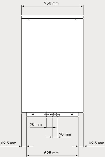
Geräteseite
