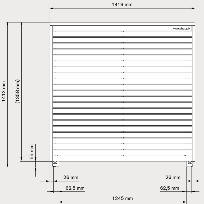
Gerätefront
