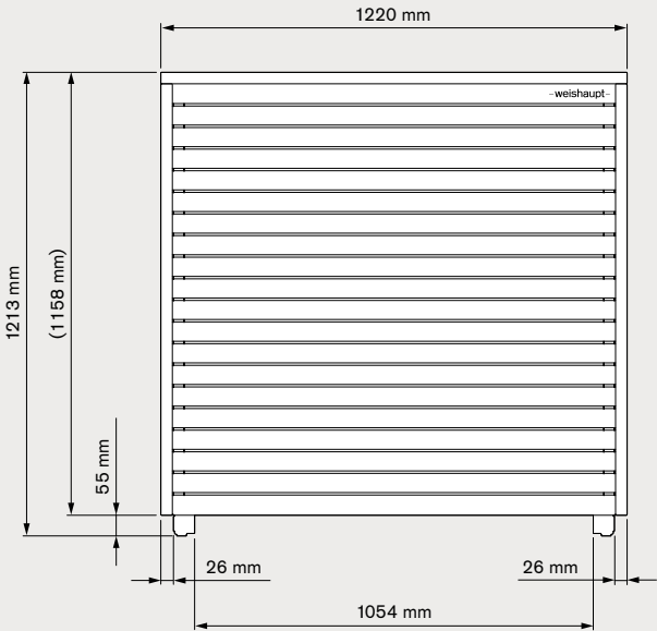
Gerätefront
