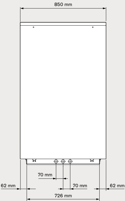
Geräteseite
